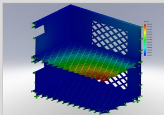
Styrkeberegningsanalyse, Finite Element Modelling (FEM)
